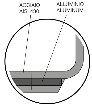
Fondo termodiffusore Thermal diffusion bottom
